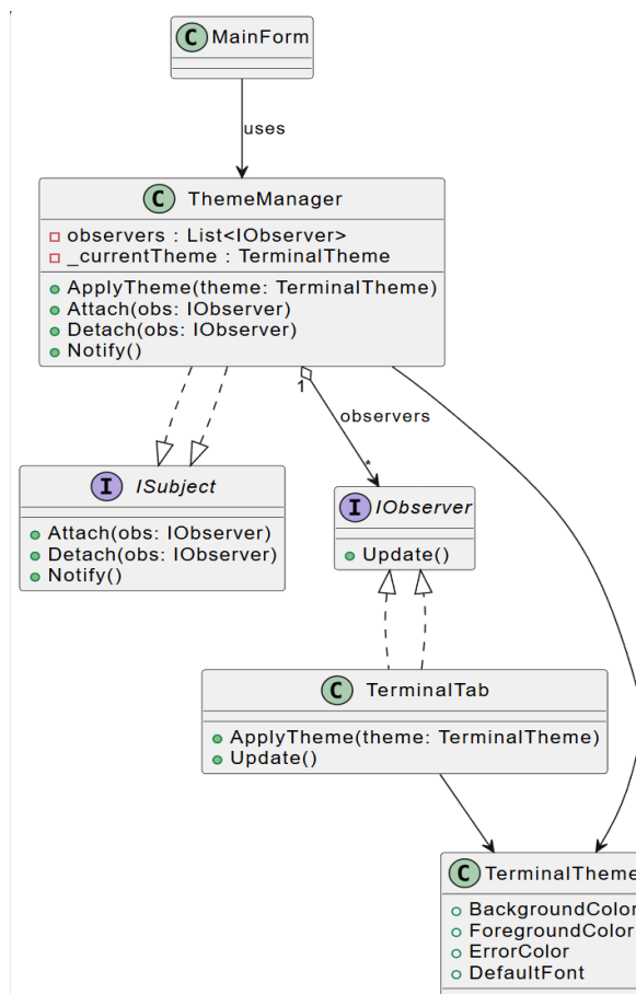
Рис 1: ClassDiagram (Observer)
